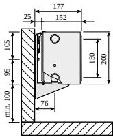
Plint, typ 33 z zawieszieniami ściennymi Monclac, widok z boku
