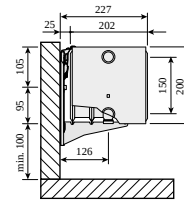
Plint, typ 44 z zawieszieniami ściennymi Monclac, widok z boku
