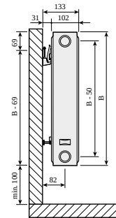
Compact, typ 22 z zawieszzeniami ściennymi, widok z boku
