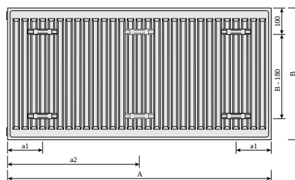
Hygiene, widok z tyłu
